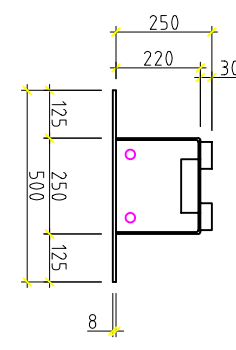
TYPSEKTION 250:250/500x8/70x30
