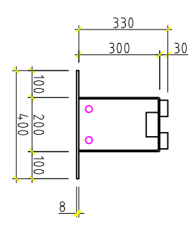
TYPSEKTION 330:200/400x8/60x30
