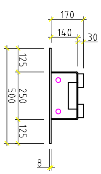
TYPSEKTION 170:250/500x8/70x30
