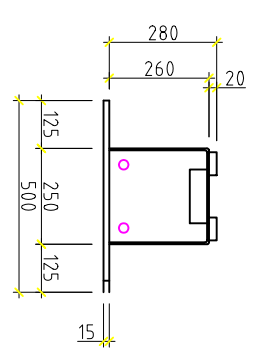
TYPSEKTION 280:250/500x15/60x20
