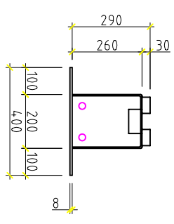
TYPSEKTION 290:250/500x8/60x30
