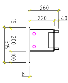
TYPSEKTION 260:200/315x8/15x4.0
