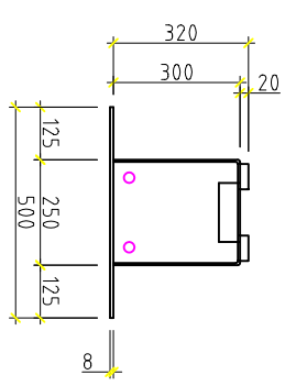
TYPSEKTION 320:250/500x8/60x20
