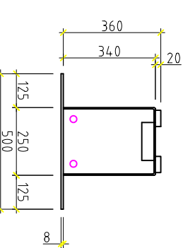
TYPSEKTION 360:250/500x8/60x20
