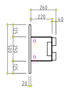
TYPSEKTION 260:250/500x20/80x4.0
