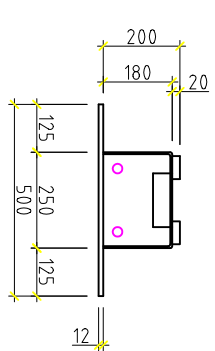
TYPSEKTION 200:250/500x12/60x20
