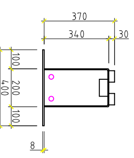
TYPSEKTION 370:200/400x8/60x30
