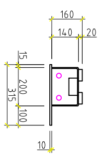
TYPSEKTION 160:200/315x10/60x20
